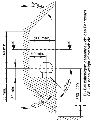
Seitenansicht
